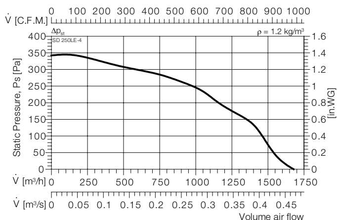
SD 250LE-4
