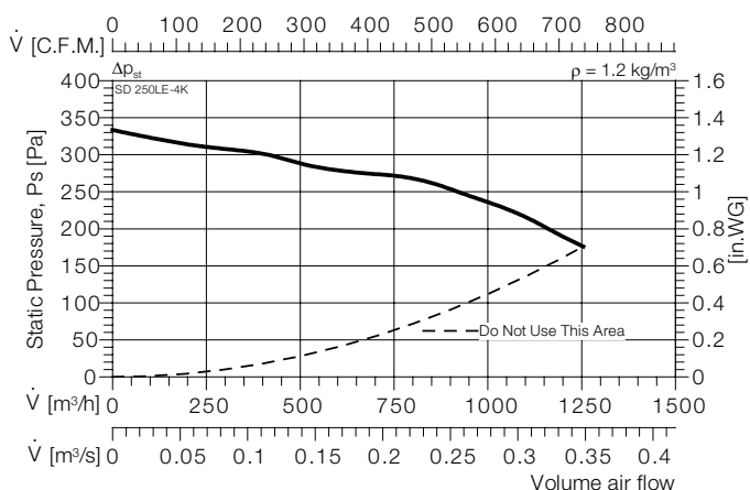
SD 250LE-4K
